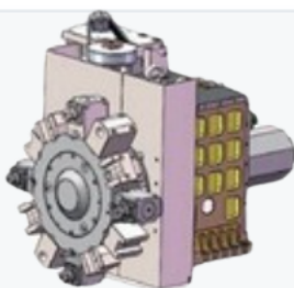
Приводна револьверна головка з віссю Y
